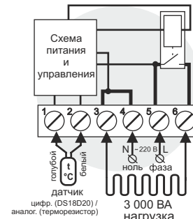
Схема 1. Упрощенная внутренняя схема и схема подключения
